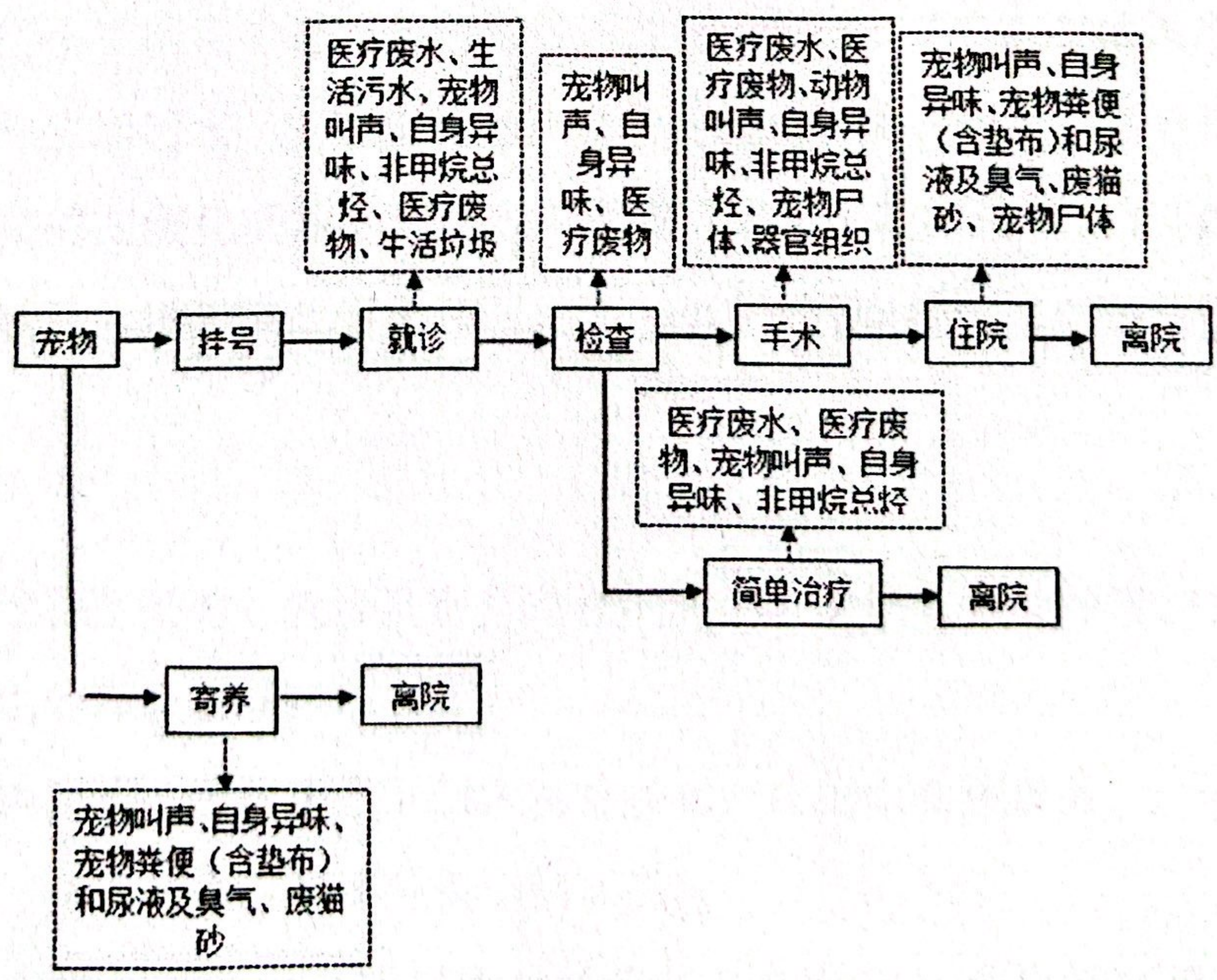
图1 营运期就诊流程及产污流程图
