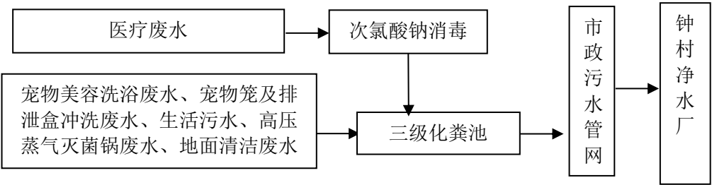
图 4-4 废水处理工艺流程图
