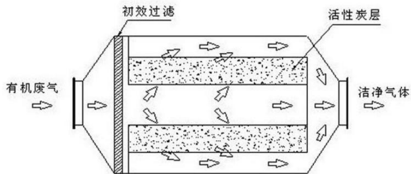
图 4-1-2 活性炭吸附装置结构图
