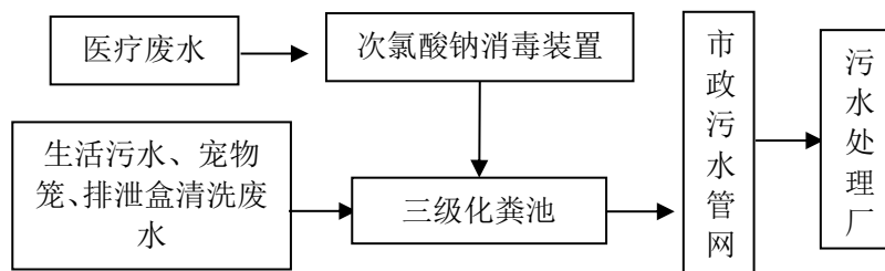
图 4-2 废水处理工艺流程图
