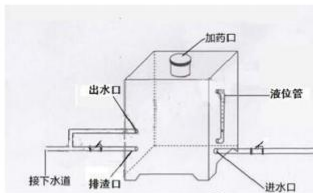
图4-2-2 项目废水消毒设备示意图
