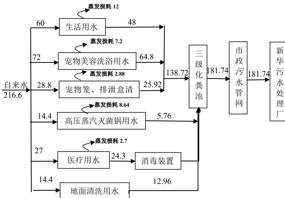
图 2-1 本项目水平衡图（单位：m³/a）
