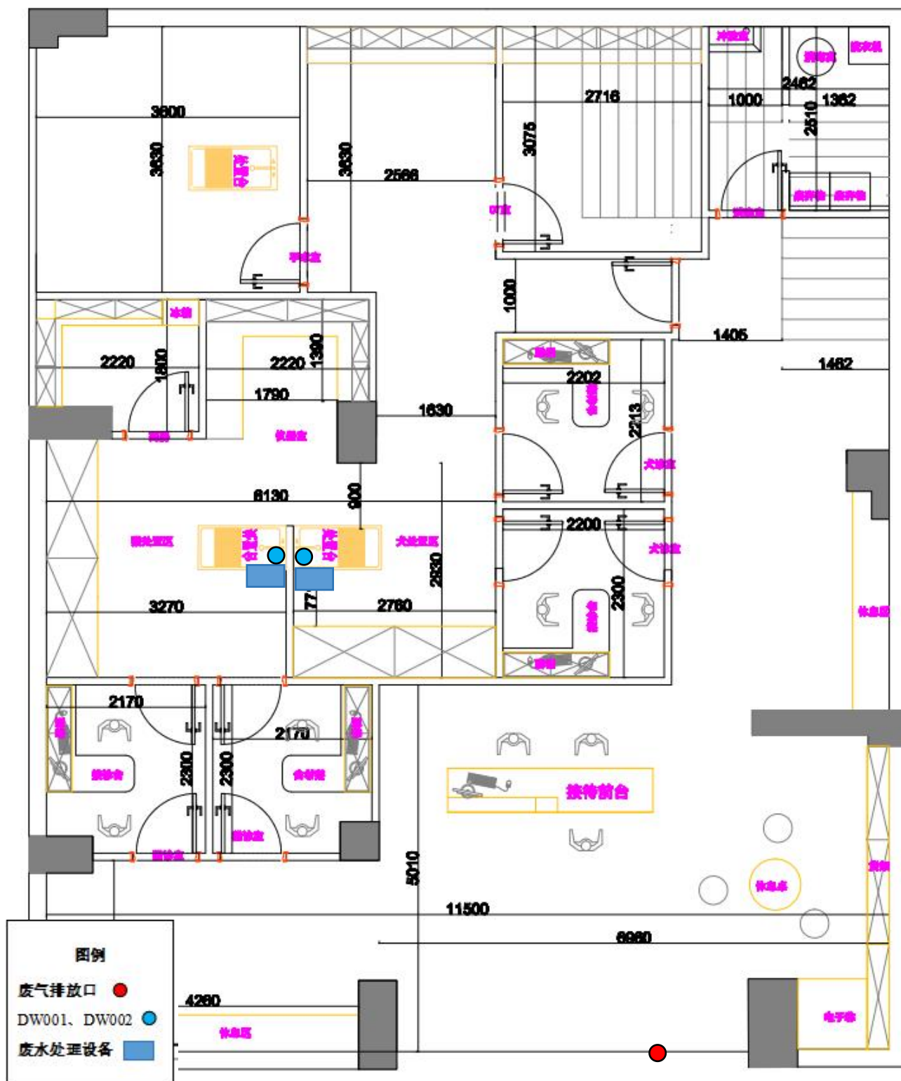
一楼平面图
