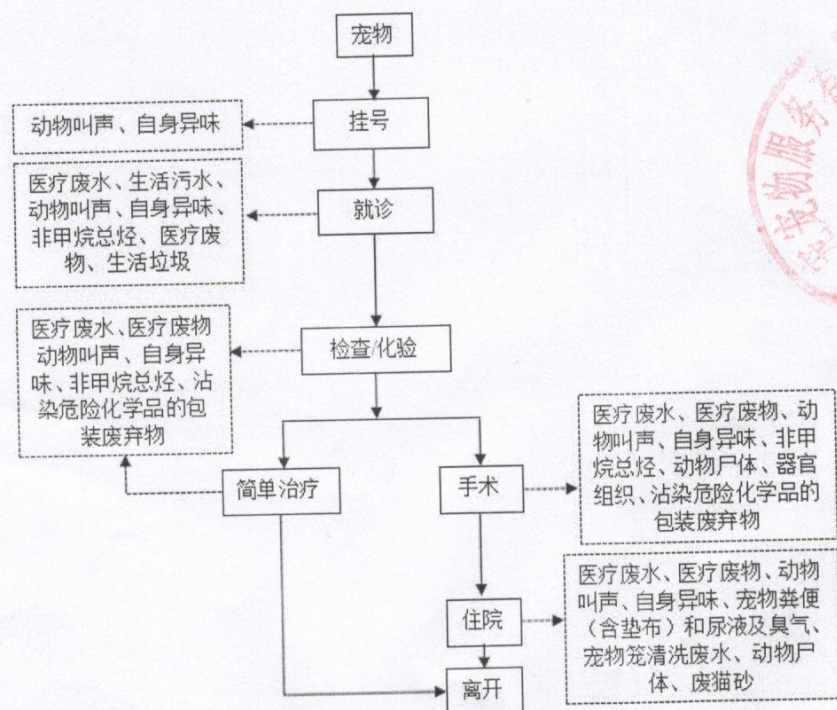
图1 营运期就诊流程及产污流程图
