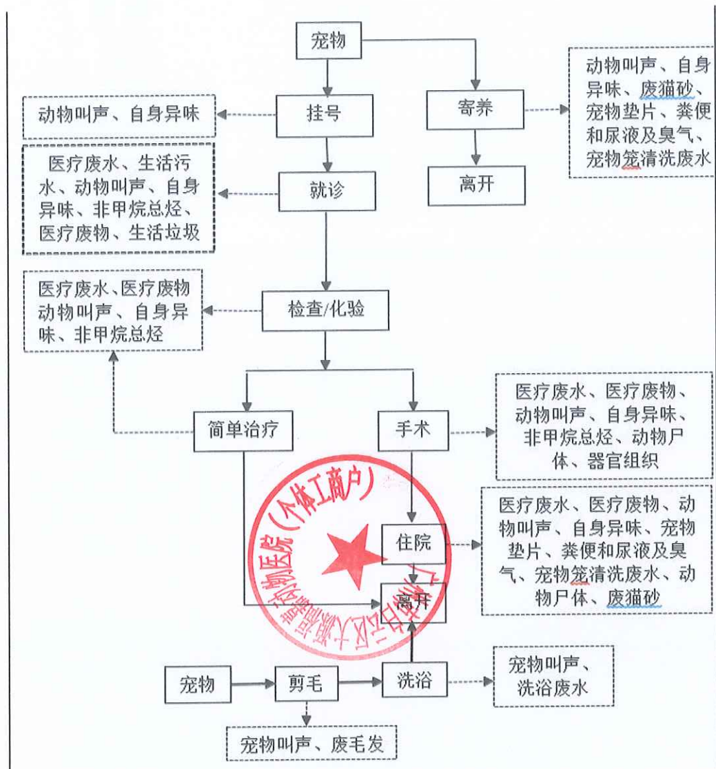
图1 营运期工艺流程及产污流程图
