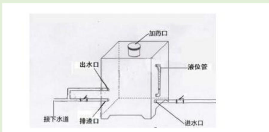
图4-2 项目废水消毒设备示意图
