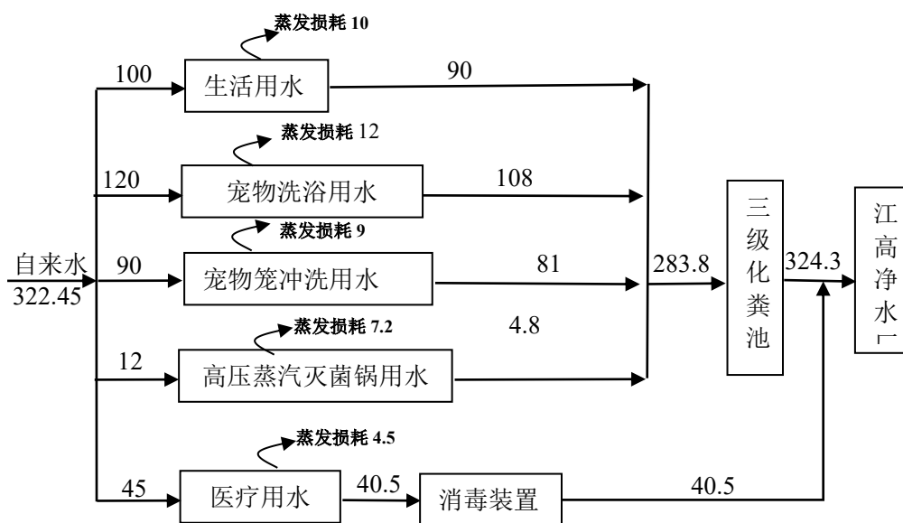
图 2-1 本项目水平平衡图 (单位: \text{m}^3/\text{a} )
