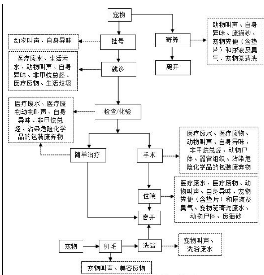
图1 营运期工作流程及产污流程图
