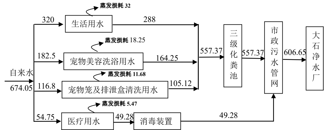
图 2-1 项目水平衡图 (m 3 /a)
