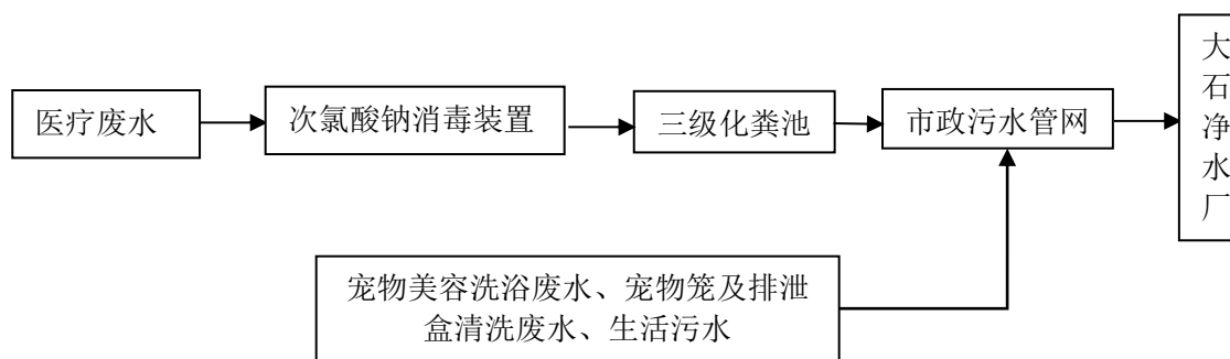
图4-2 废水处理工艺流程图
