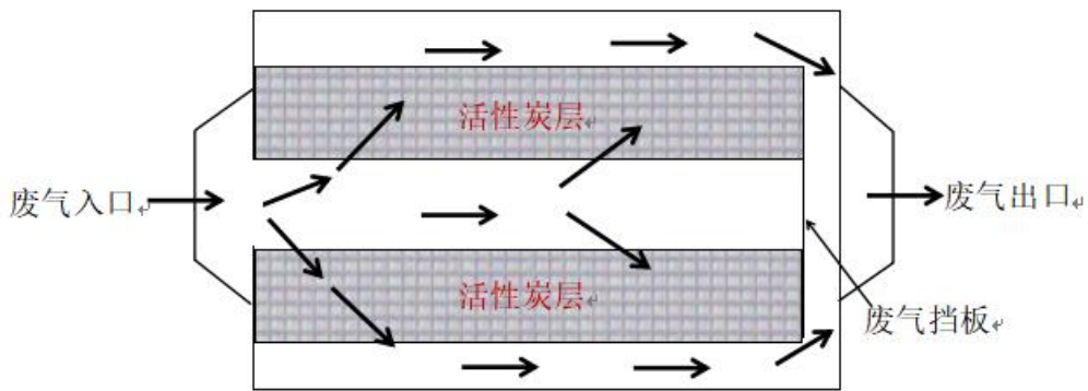
图 4-1 活性炭装置示意图
