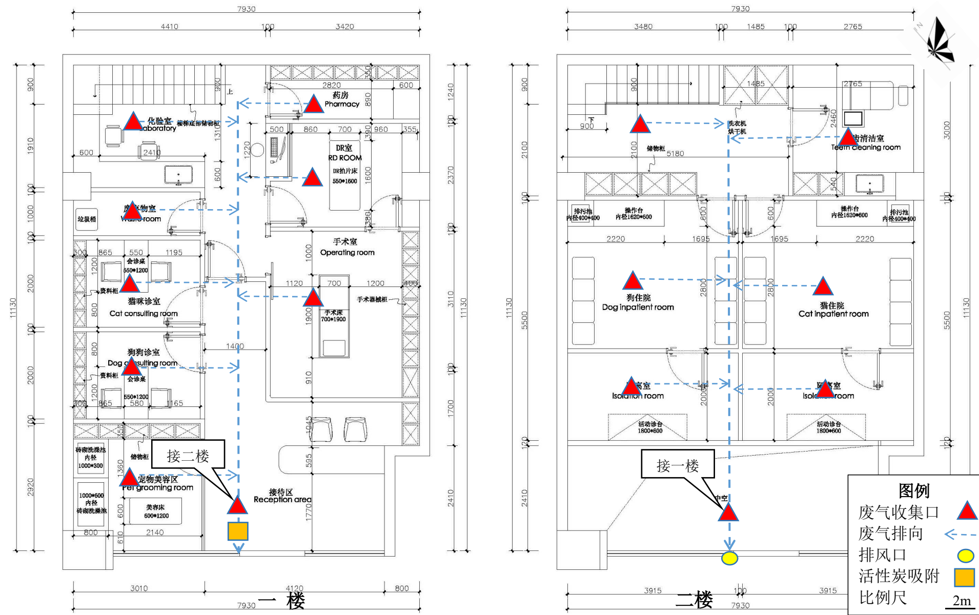
附图 4-1 项目平面布置及废气流向图
