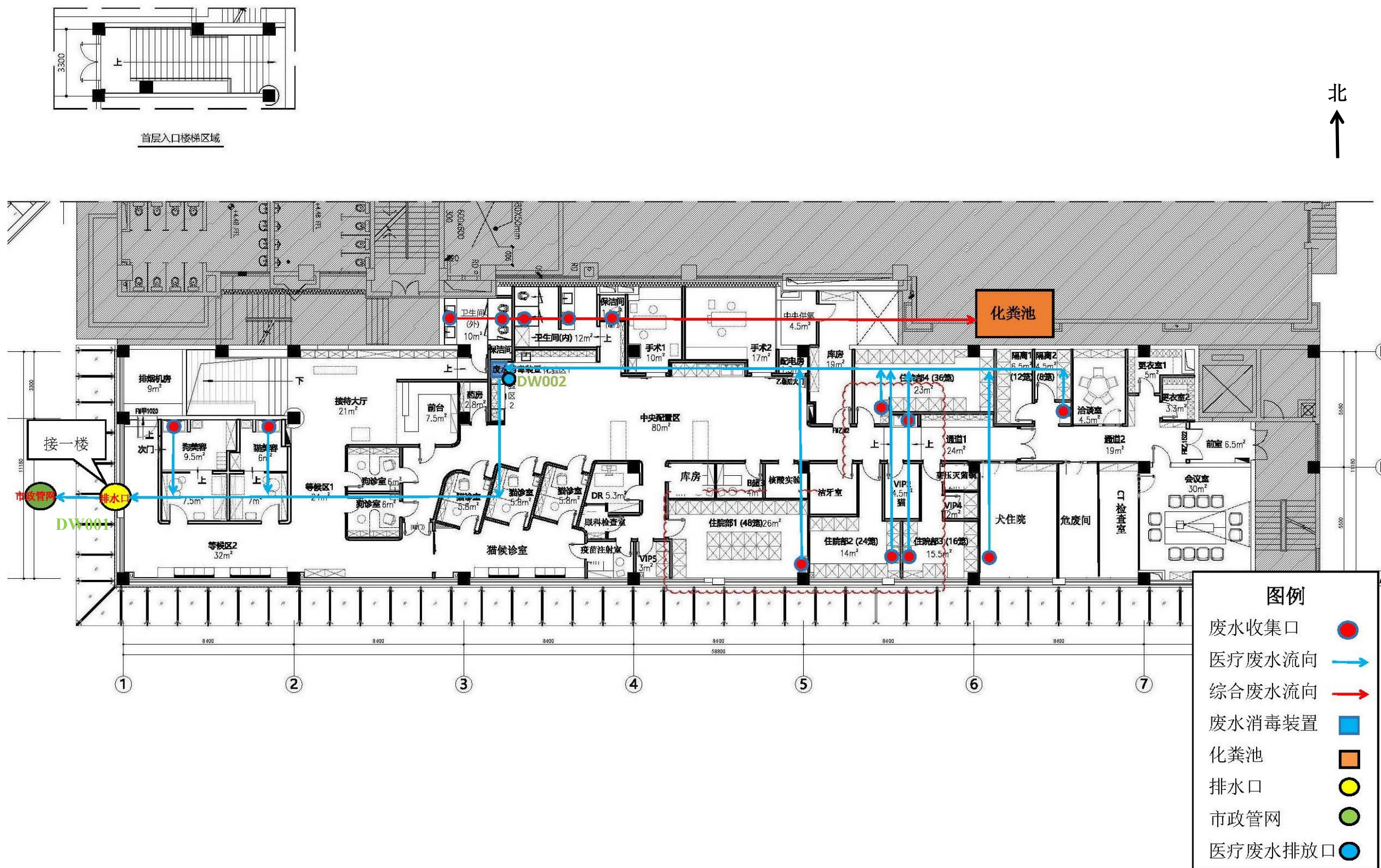
附图 4-3 项目平面布置图-排水图
