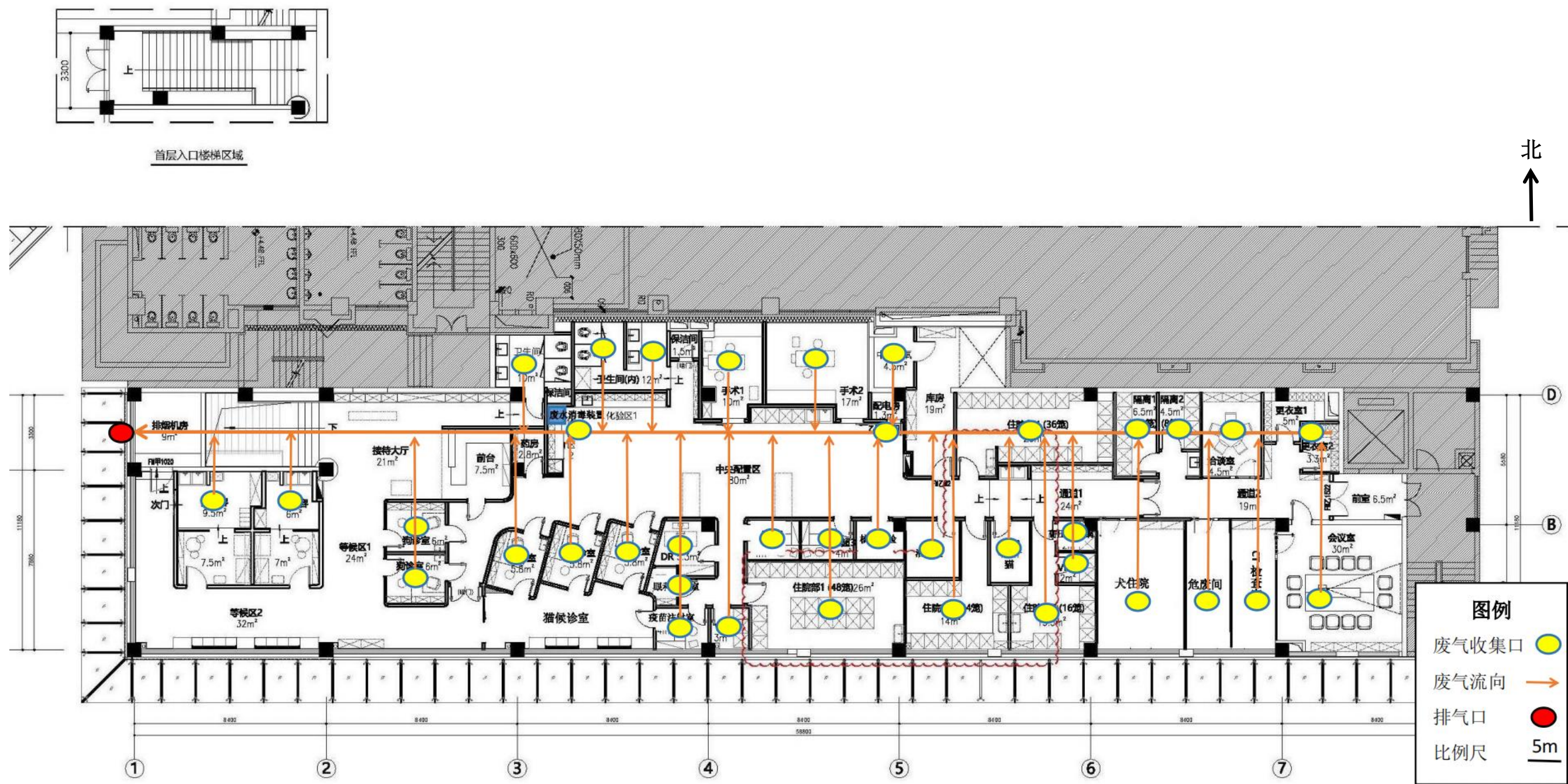
附图 4-2 项目平面布置图-排气图
