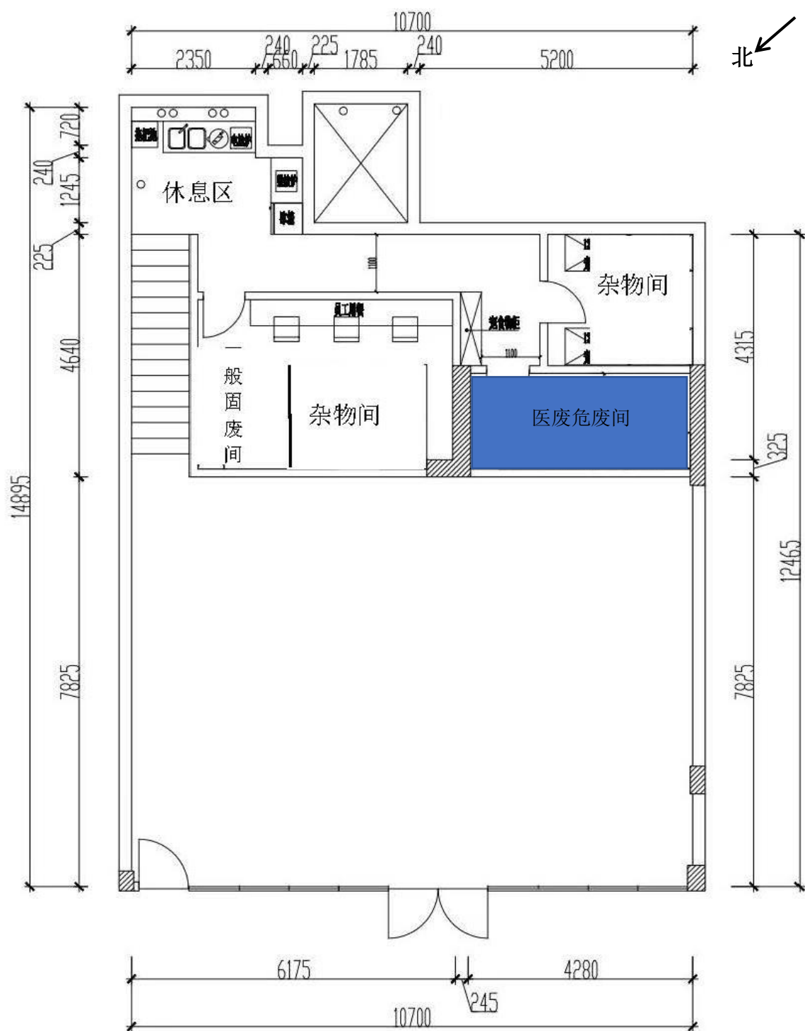
附图 4-2 项目二楼（夹层）平面布置图
