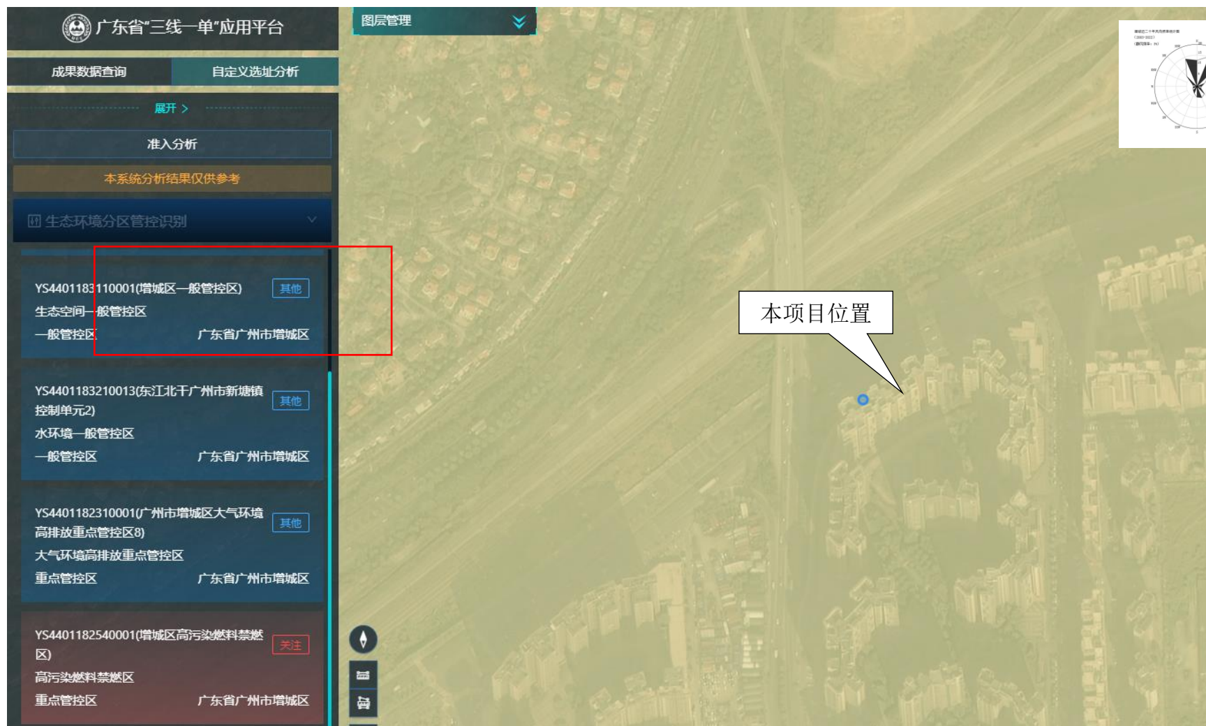
附图 18 广东省“三线一单”应用平台-生态空间一般管控区
