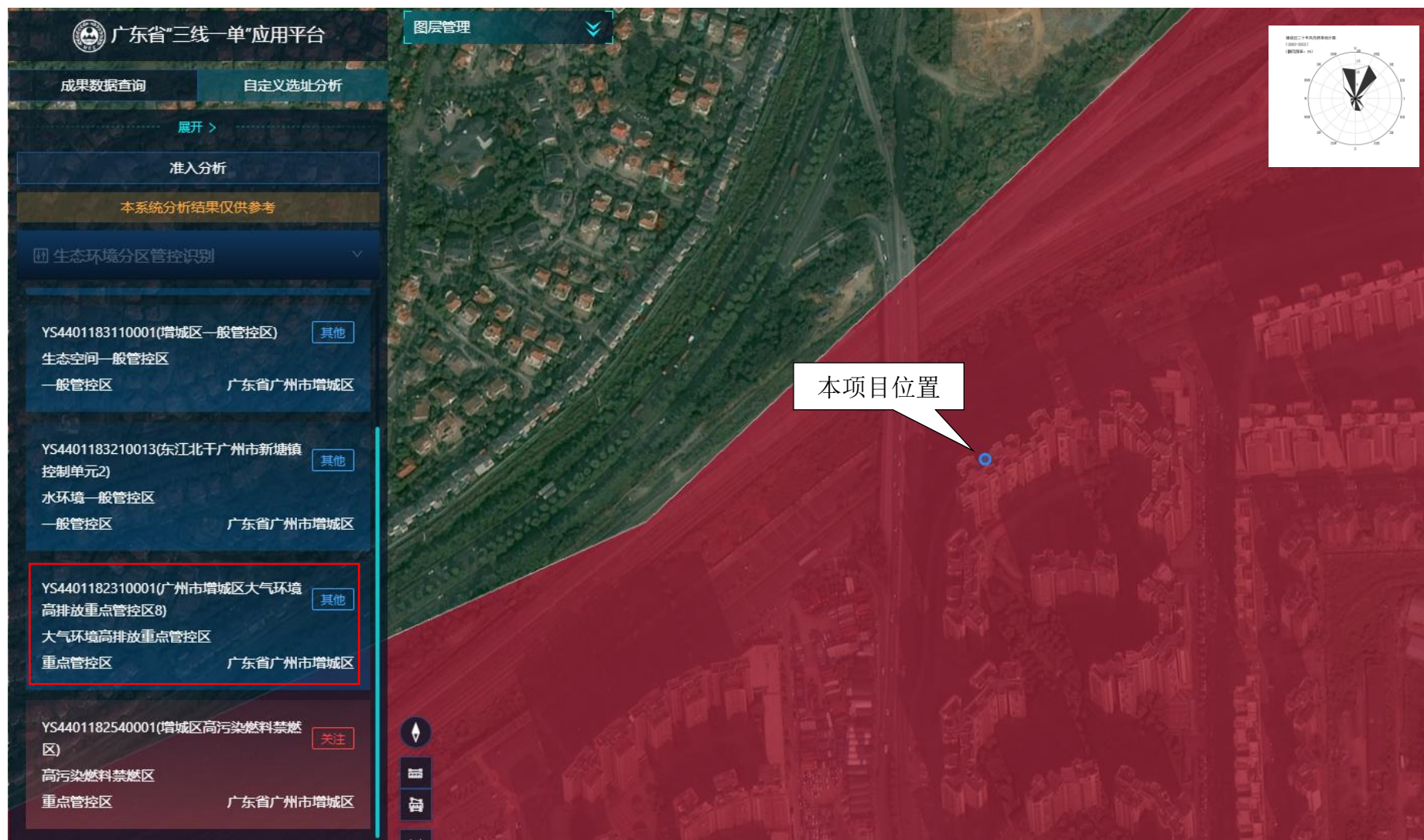
附图 16 广东省“三线一单”应用平台-大气环境受体敏感重点管控区截图
