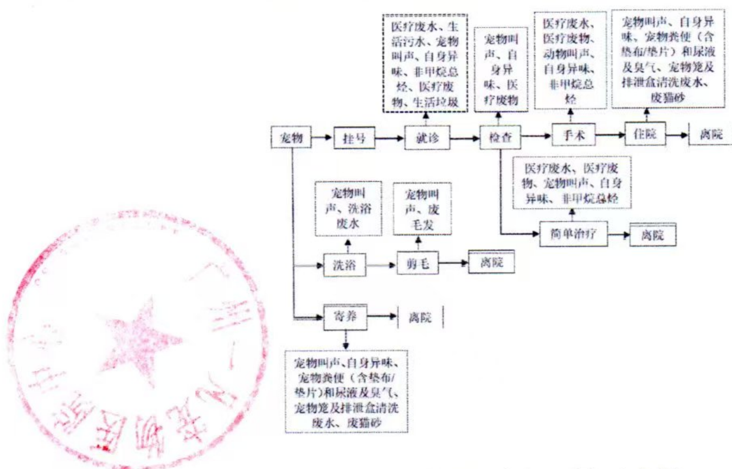
图 1 营运期工艺流程及产污流程图
