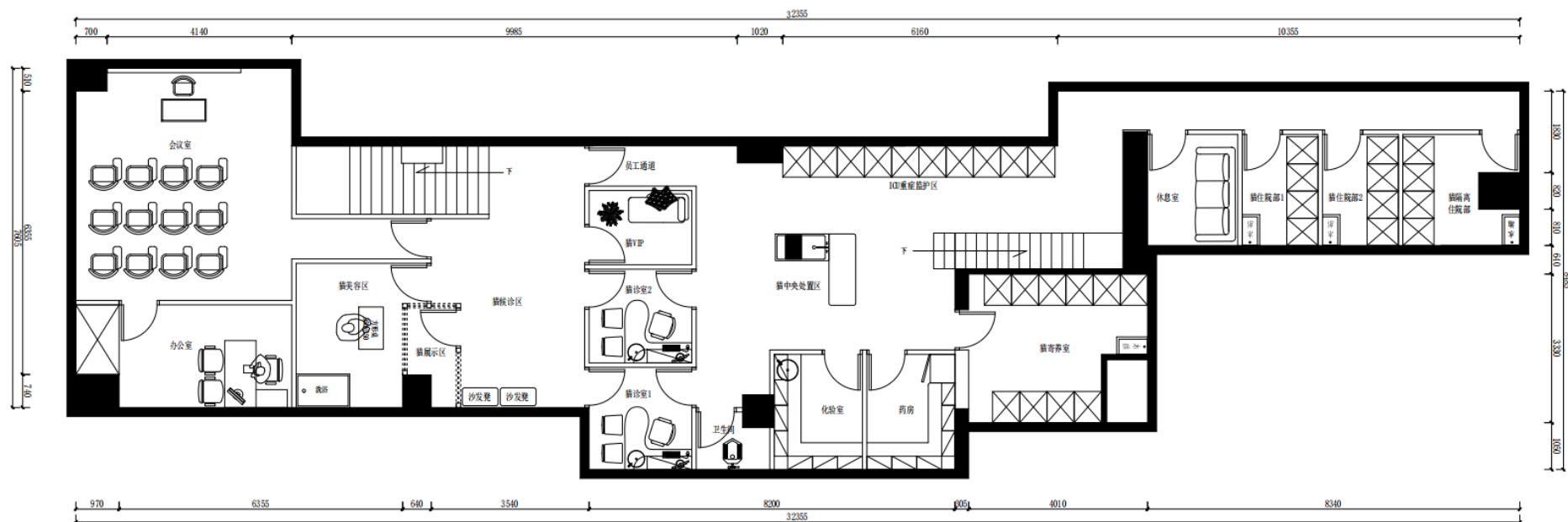
二层平面布局图 比例1:90
