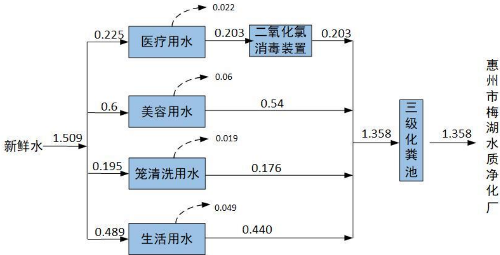
图 2-1 项目运营期水平衡图 单位：t/d
