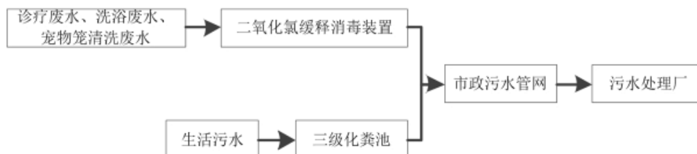
图 4-1 综合废水处理工艺流程图
