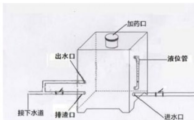
图 4-2 项目综合废水消毒设备示意图
