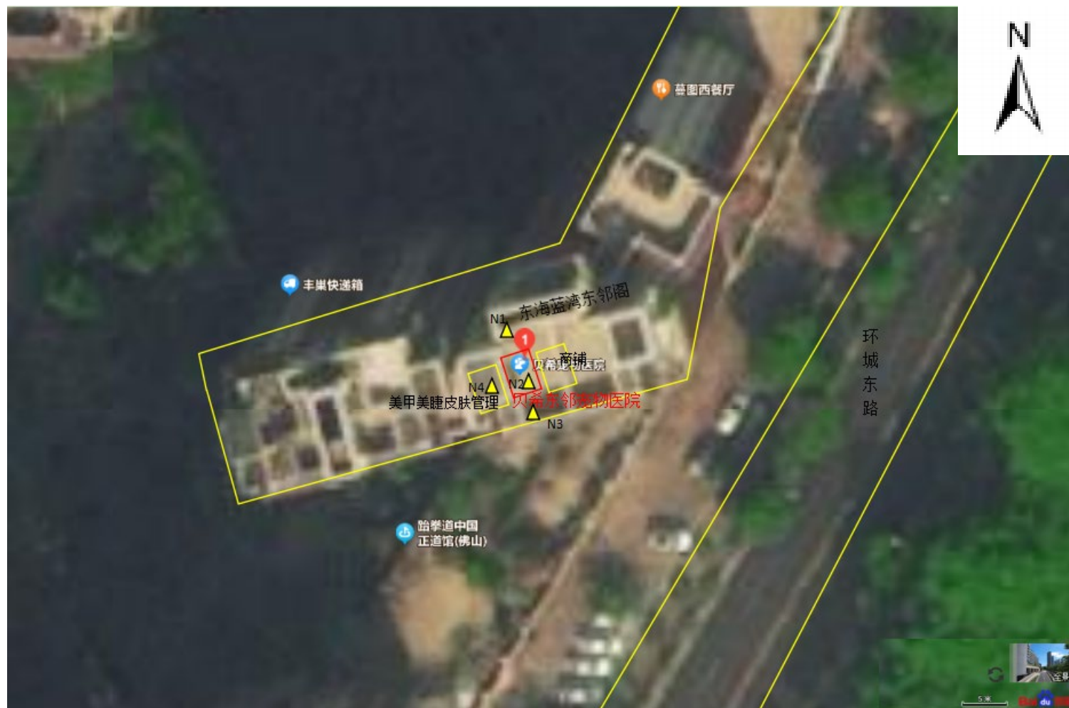
附图 5 声环境现状监测点位图
