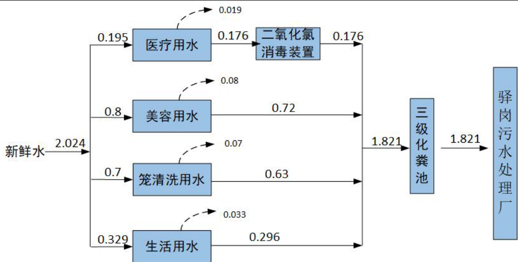
图 2-1 项目水平衡图 (m³/d)
